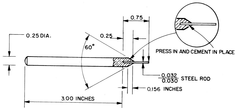
Loctite Applicator P/N 2550982
